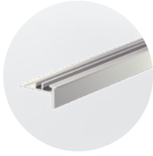
Profil Incizo/ Hliníkový dílčí schodový profil Incizo QSVINCP(-) / NEVINCPBASE1 2 000 x 45 x 8 mm / 2 000 x 33 x 17 mm
